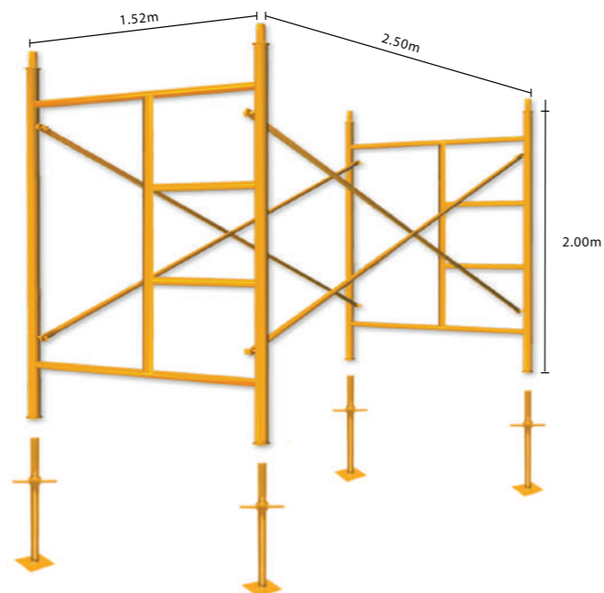
Andamio Amplio
