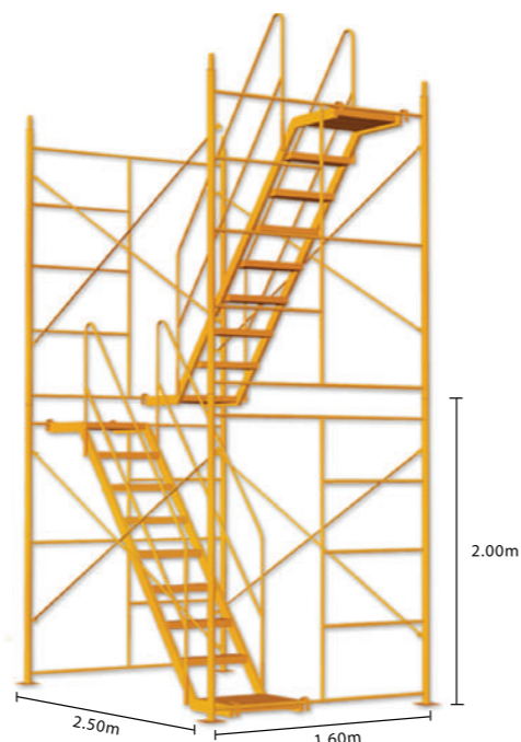
Módulo Escalera
